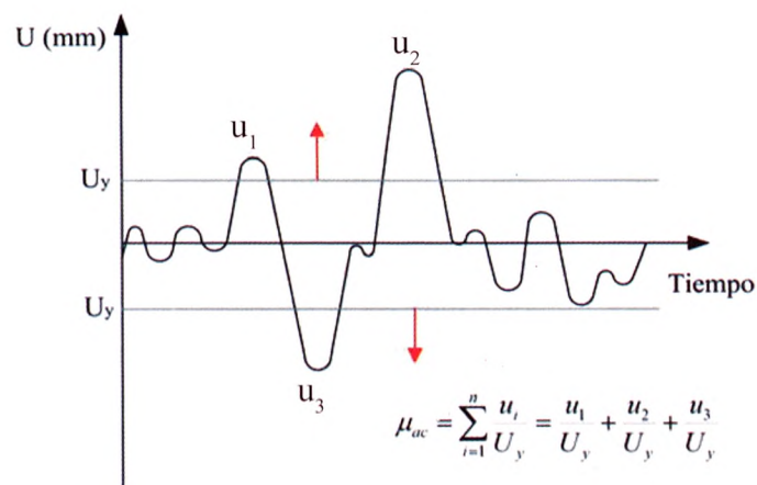
Figura 6: Evaluación de la ductilidad acumulada \mu_{ac}
