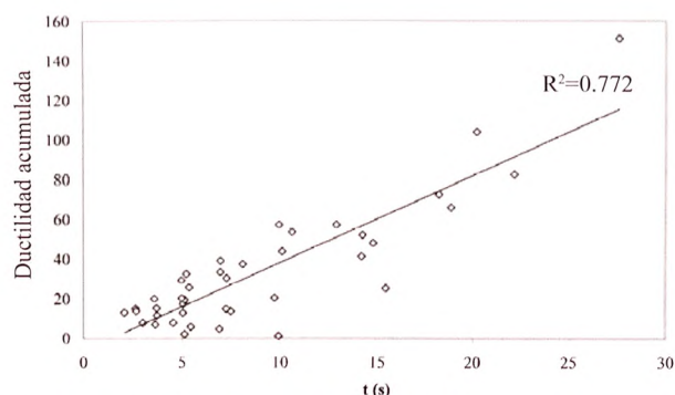
Figura 12: Relación ductilidad acumulada versus duración
