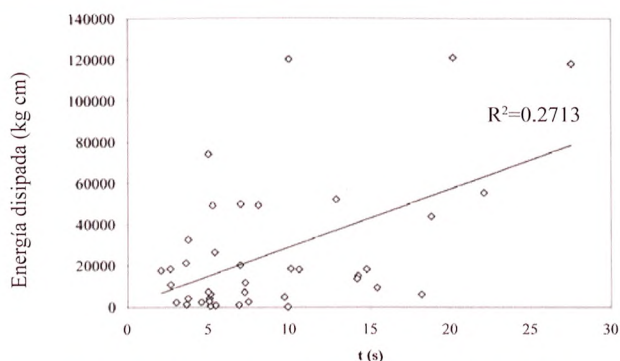
Figura 11: Relación energía disipada versus duración
