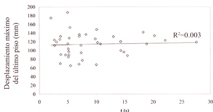
Figura 10: Relación desplazamiento máximo del último piso versus duración
