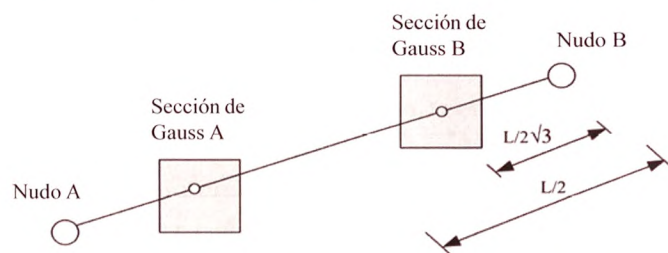
Figura 1: Secciones de Gauss a lo largo de la longitud de un miembro de hormigón armado
