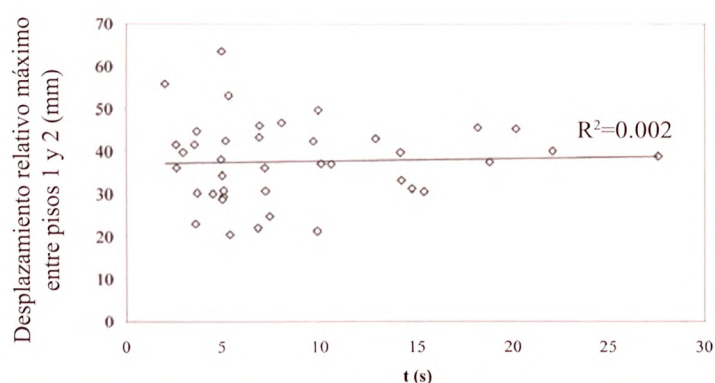
Figura 9: Relación desplazamiento máximo relativo versus duración
