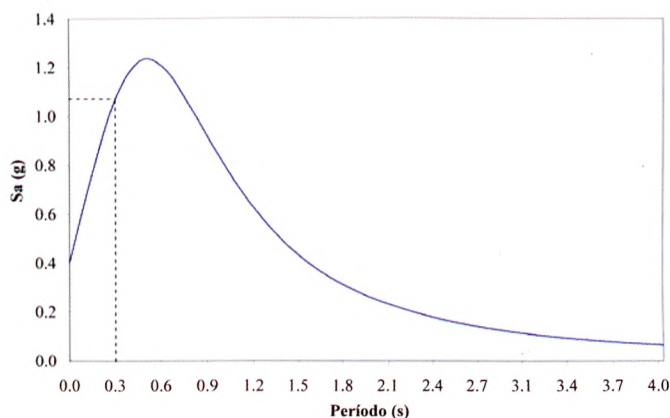
Figura 5: Espectro de diseño utilizado en este estudio propuesto por la norma NCh433 Of.96
