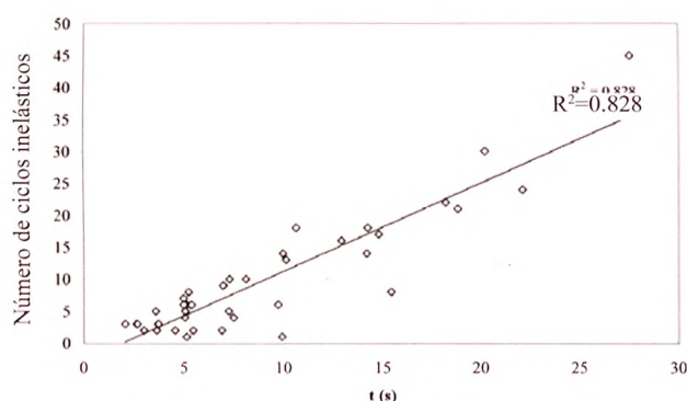
Figura 13: Relación número de ciclos inelásticos versus duración
