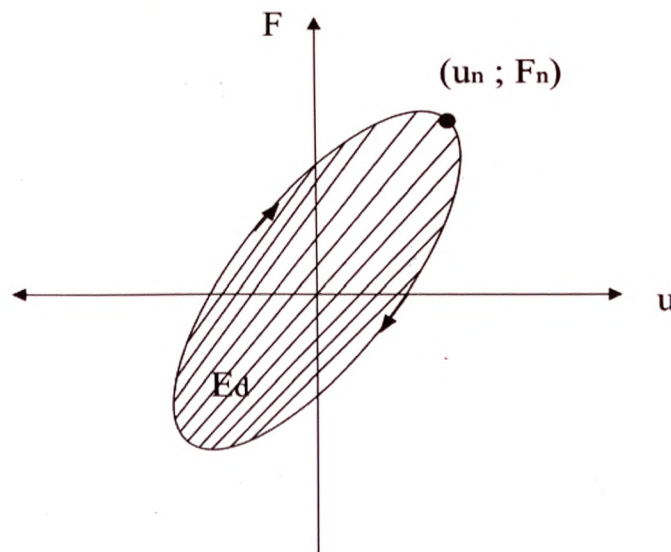
Figura 7: Evaluación de la energía de histéresis disipada
